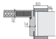
P 005 DÜZ KASA STANDART
