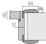
P 108 DÜZ KASA OPSIYONEL
