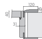
P 808 EKO KASA OPSİYONEL
