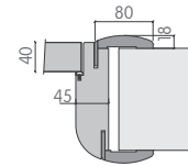
P 108 / 107 BOMBE DÜZ KASA OPSİYONEL
