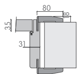
P 208 EKO KASA STANDART
