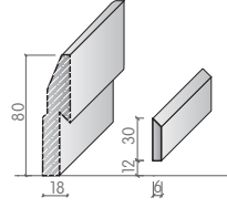
808 SÜPÜRGELİK H:80mm D:18mm Aski Sistem
