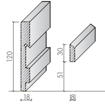
005 SÜPÜRGELİK H:120mm D:18mm Aski Sistem
