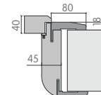
P 208, P107 BİNİLİ KASA OPSİYONEL
