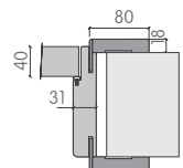
P 005 DÜZ KASA STANDART
