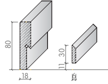
005 SÜPÜRGELİK H:80mm D:18mm Aski Sistem
