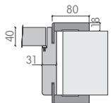
P 005 DÜZ KASA STANDART
