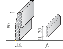
208 SÜPÜRGELİK H:80mm D:18mm Aski Sistem
