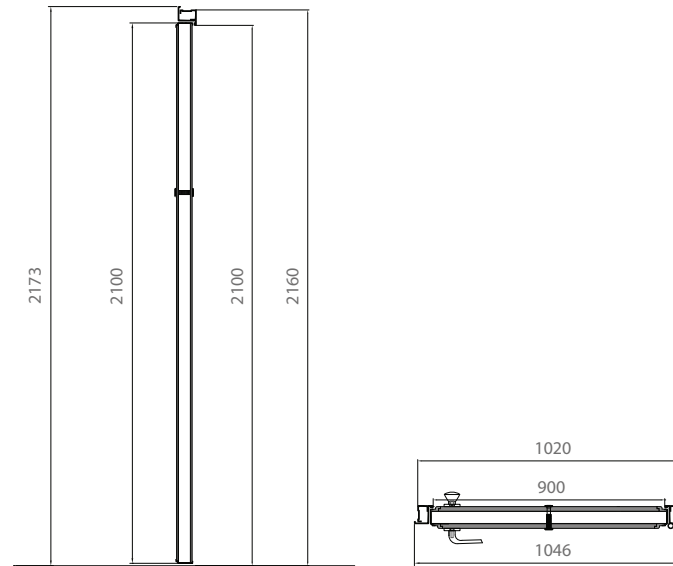
ABS panel üretim kesit
